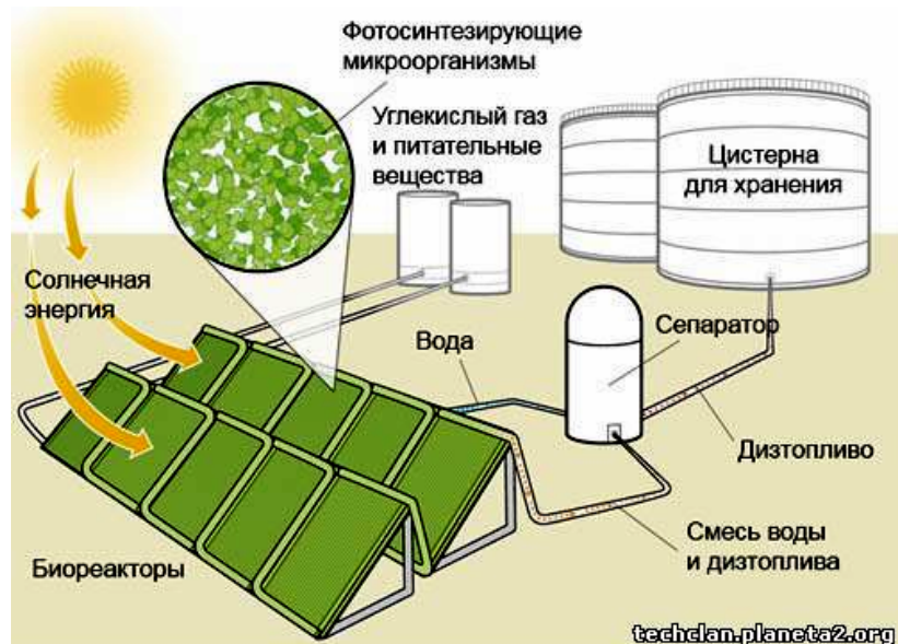
Рис. 119. Система биореакторов «топливная ферма» поглощает солнечный свет и, потребляя углекислый газ и питательные вещества, производит биотопливо в ходе фотосинтеза.
