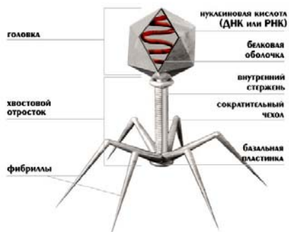
Рис. 111. Внешний вид (верхняя часть рисунка) и схема строения (нижняя часть рисунка) бактериофага (описание в тексте)
