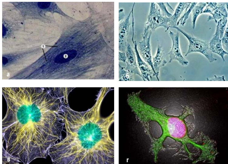
Рис. 6. Фибробласты. Изображения получены с помощью: а) световой микроскопии (1 – актиновые микрофиламенты, 2 – ядро), увеличено в 1000 раз, \times 1000 ; б) фазово-контрастной микроскопии, \times 500 ; в) иммунофлуоресцентной микроскопии (микротрубочки окрашены в желтый цвет, актиновые микрофиламенты – голубой, ядро – зеленый), \times 980 ; г) конфокальной микроскопии, \times 1000
