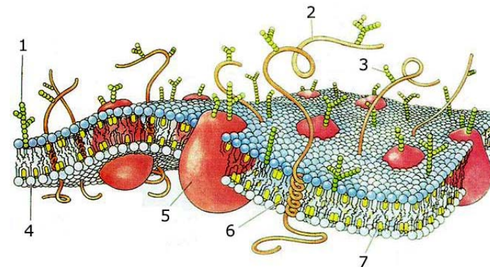
Рис. 36. Мембранные рецепторы в структуре клеточной мембраны (плазмалеммы). 1 – углеводы, связанные с липидами мембраны (гликолипиды); 2 – свободные концы рецепторов гликопротеиновой природы; 3 – «антенны»; 4 – гидрофильные участки бимолекулярного слоя липидов; 5,6 – рецепторы; 7 – гидрофобные участки бимолекулярного слоя липидов
