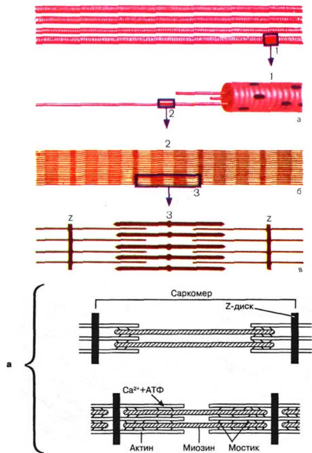
Рис. 39. Схема мышечного сокращения, в котором участвует белковый мотор линейного движения на основе белка миозина: 1 – мышечное волокно; 2 – фрагмент специального органоида мышечного волокна – миофибриллы; 3 – молекулы миозина; на нижней (черно-белой) части рисунка показана ½ цикла прямолинейного перемещения молекул миозина по отношению к молекулам актина так, что степень взаимного «перекрывтия» молекул с образованием временных связей (мостиков) увеличивается
