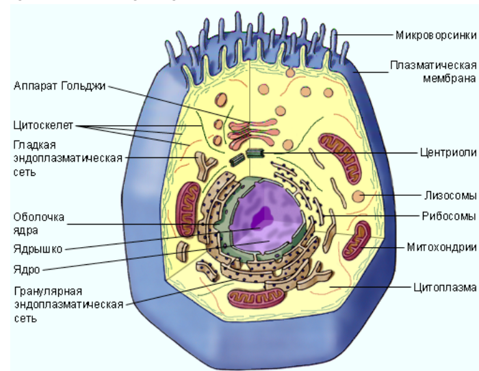
Рис. 76. Мембранные и немембранные органоиды животной клетки (описание в тексте)
