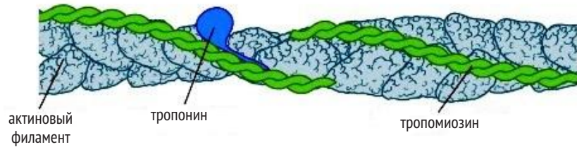
Рис.88. Актиновый микрофиламент
