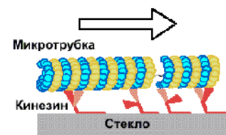
Рис. 100. Кинезиновый наноконвейер
