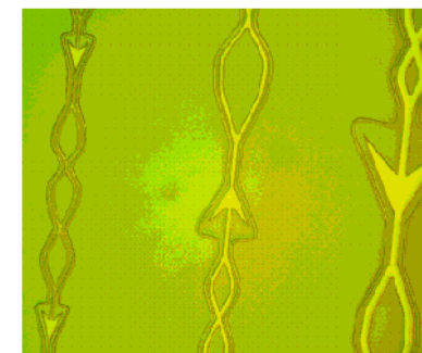
Рис. 100. Кинезиновый наноконвейер
